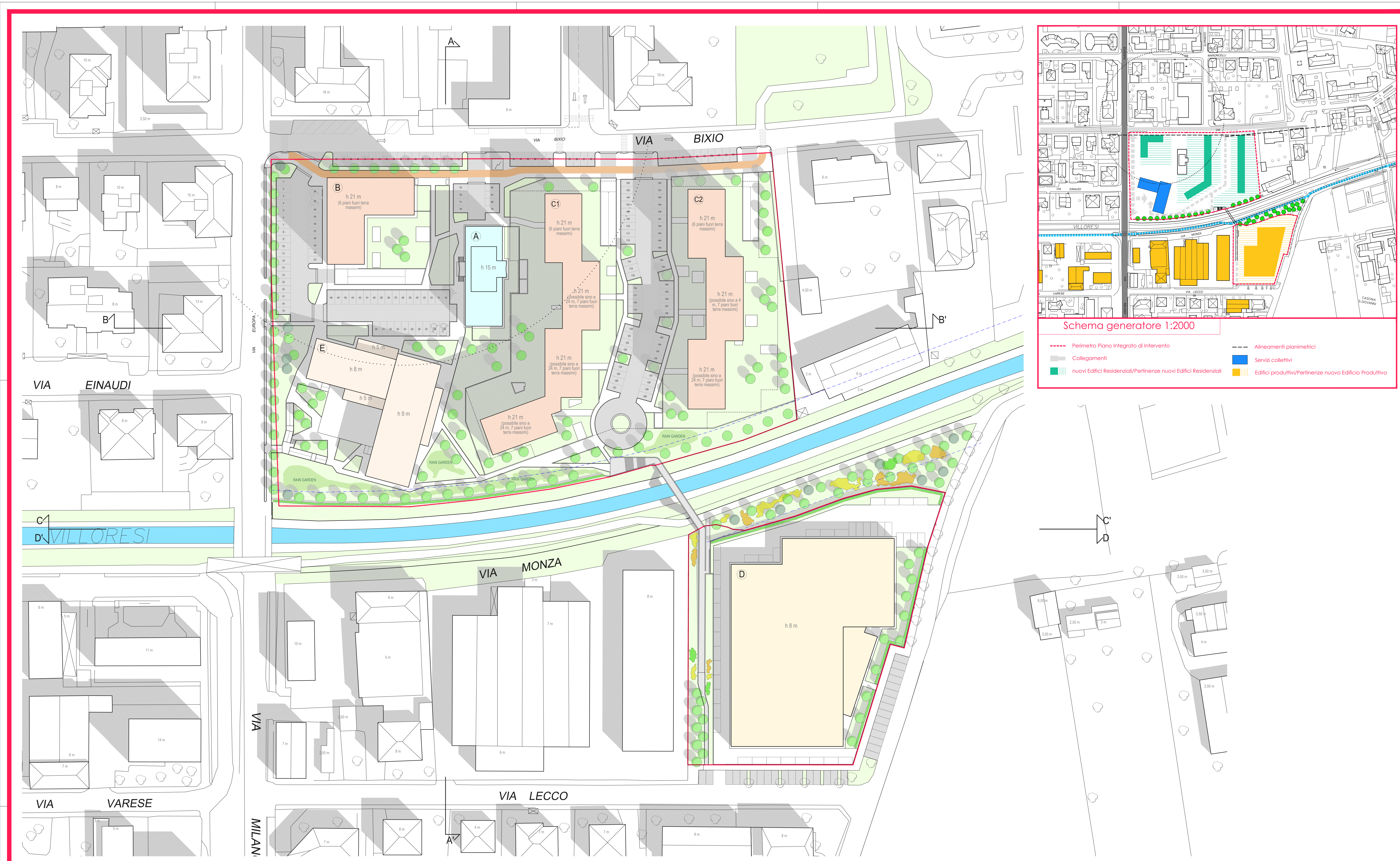
Planivolumetrico - progetto - 1:500 (con altezze "Urbanistiche" da definizione art. 3.7 NTA PR, indicative per gli edifici esistenti del contesto)
