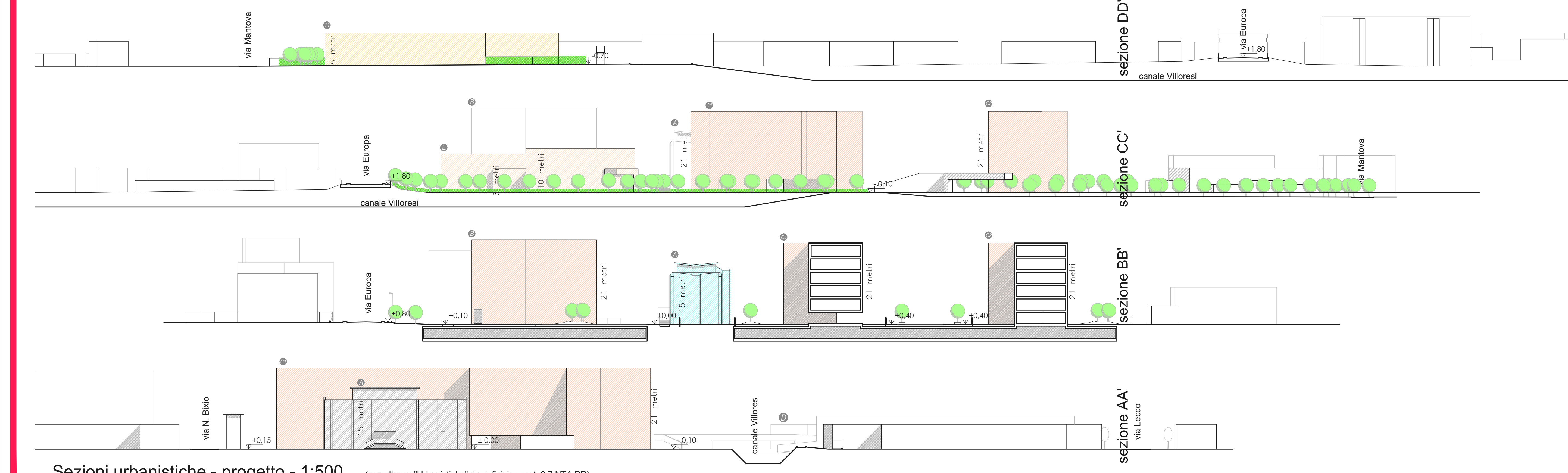
Sezioni urbanistiche - progetto - 1:500 (con altezze "Urbanistiche" da definizione art. 3.7 NTA PR)
